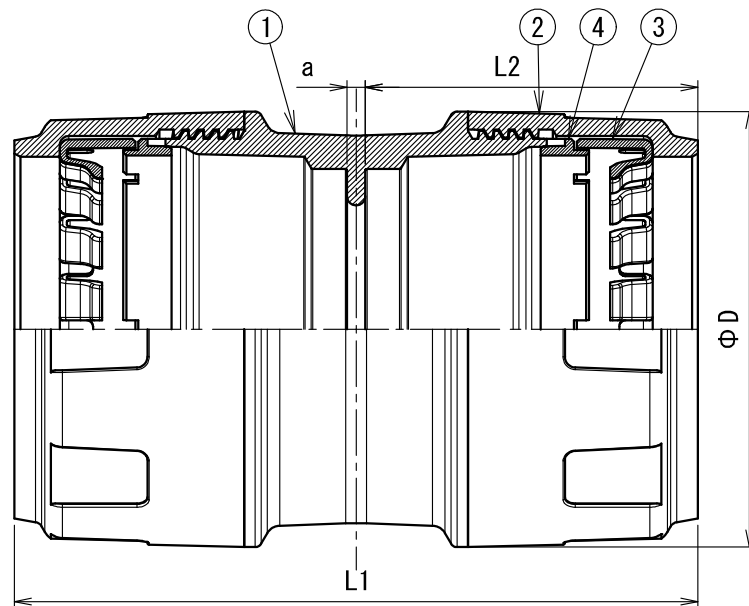
断面 A-A
